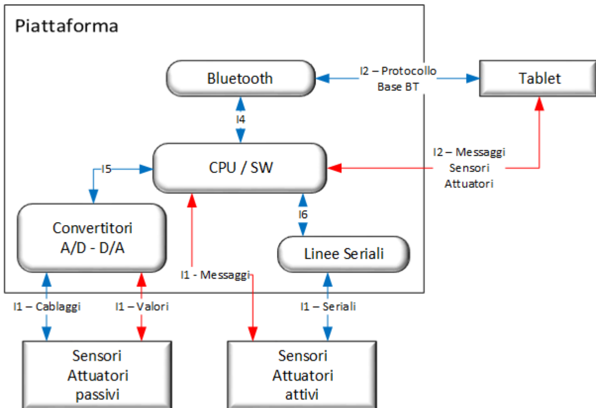
Figura 6 : Piattaforma – diagramma di contesto
