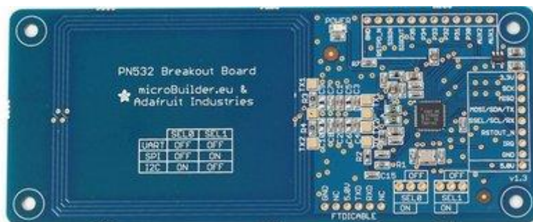
Figura 16 : Sistema locale di identificazione RFID - PN 532 RFID/ NFC (Arduino like)
