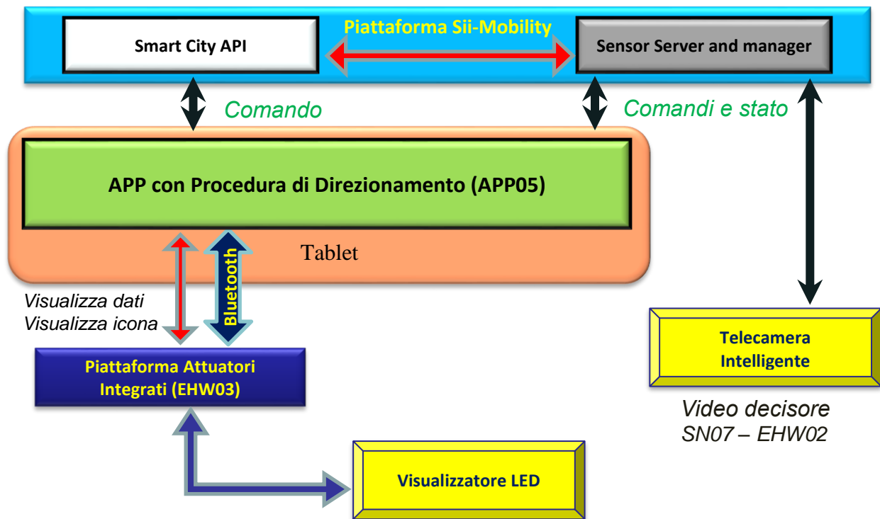
Figura 12 : Architettura generale del Direzione
