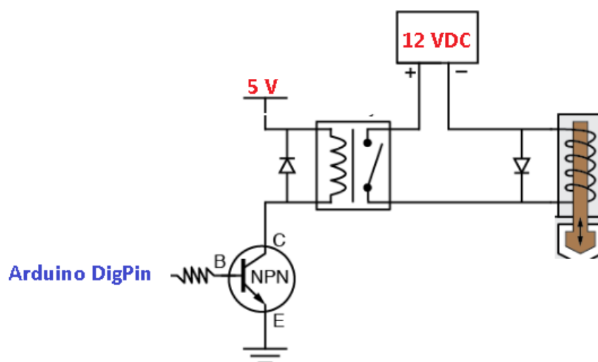
Figura 24 : schema di principio di controllo tramite pin digitale di Arduino del singolo solenoide responsabile del gancio/sgancio della bicicletta allo stallo
