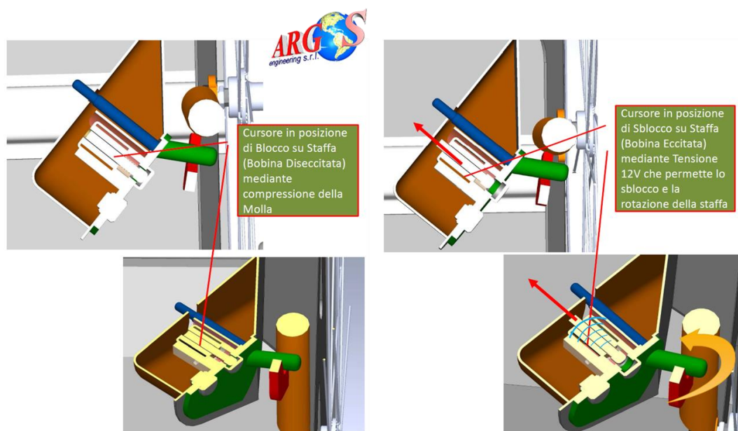
Figura 23 : cursore in posizione di blocco mediante compressione a molla (Sx) e cursore in posizione di sblocco mediante applicazione di eccitazione della bobina tramite una tensione di 12 V
