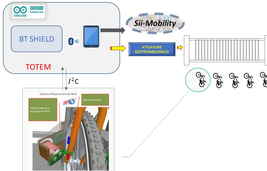
Figura 19 : Architettura generale di principio del sistema elettronico, caso operativo di rastrelliera con singolo stallo. La piattaforma TOTEM comunica con i lettori RFID tramite porta seriale I 2 C
