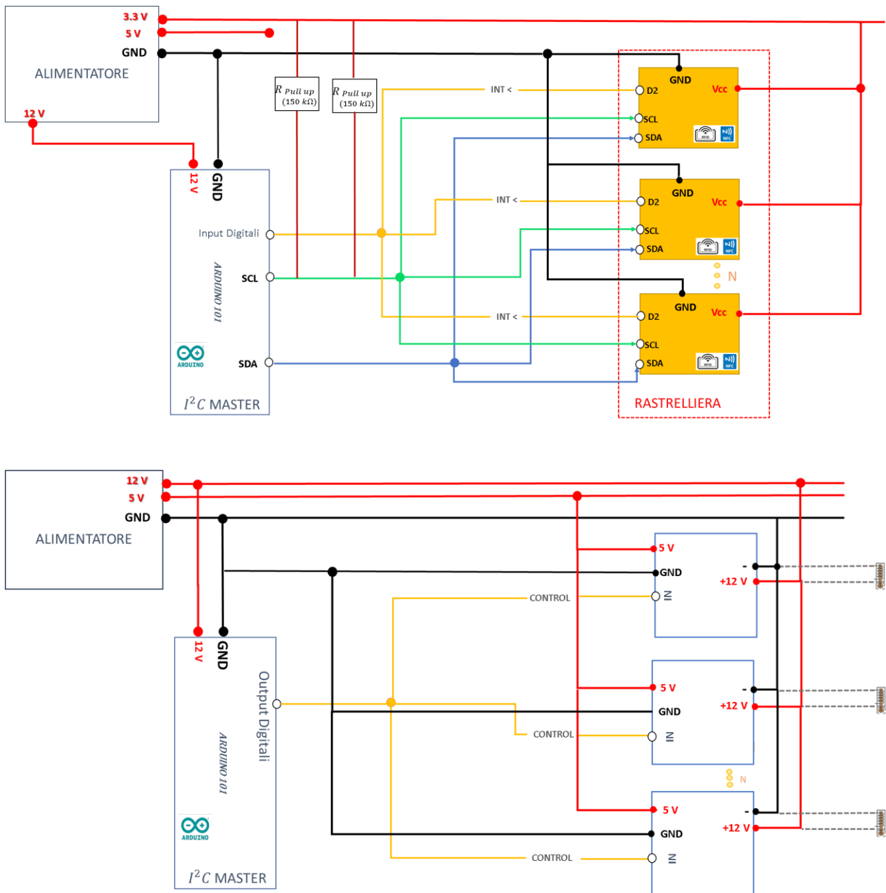
Figura 14 : Schema generale della Rastrelliera Intelligente-definizioni delle connessioni per la parte di raccolta dati proveniente dai sistemi RFID di ogni stallo(a) e comando degli attuatori a solenoide per ogni stallo (b)
