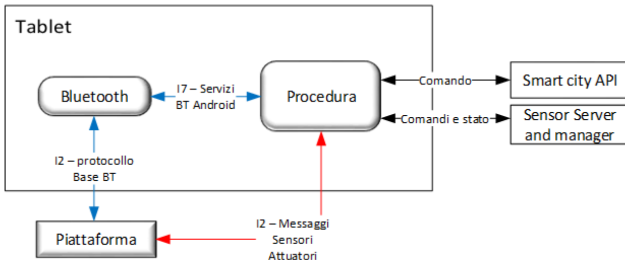
Figura 8 : Tablet – diagramma di contesto
