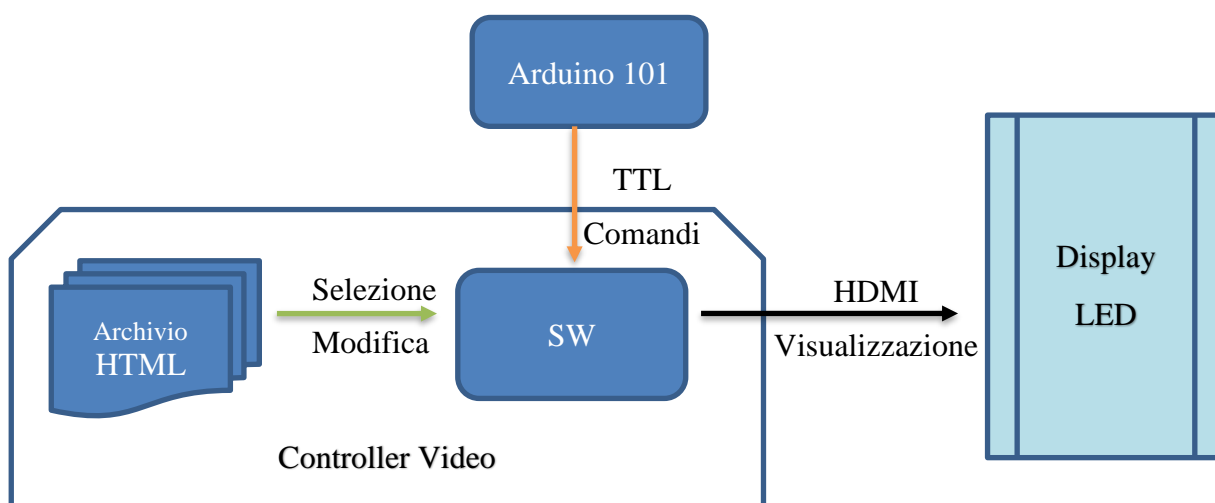
Figura 11 : Architettura del Visualizzatore LED
