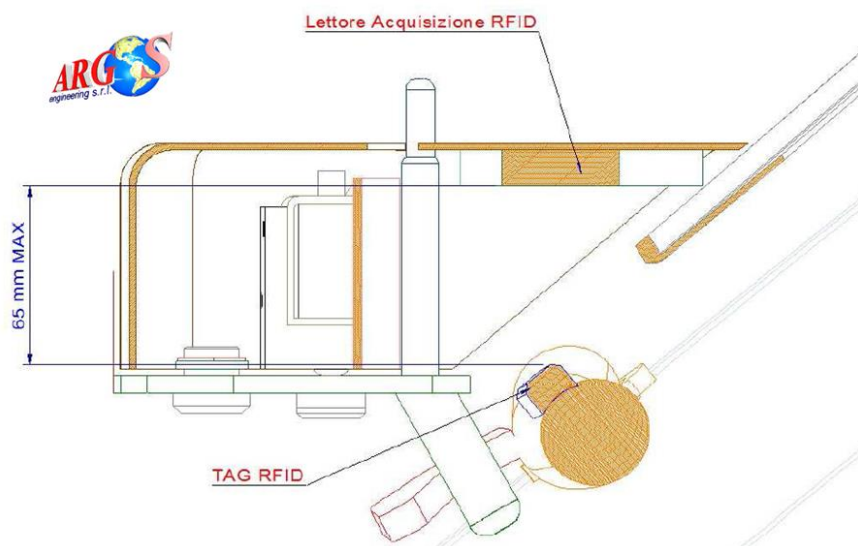
Figura 15 : Sistema locale di identificazione RFID installato sullo stallo della rastrelliera
