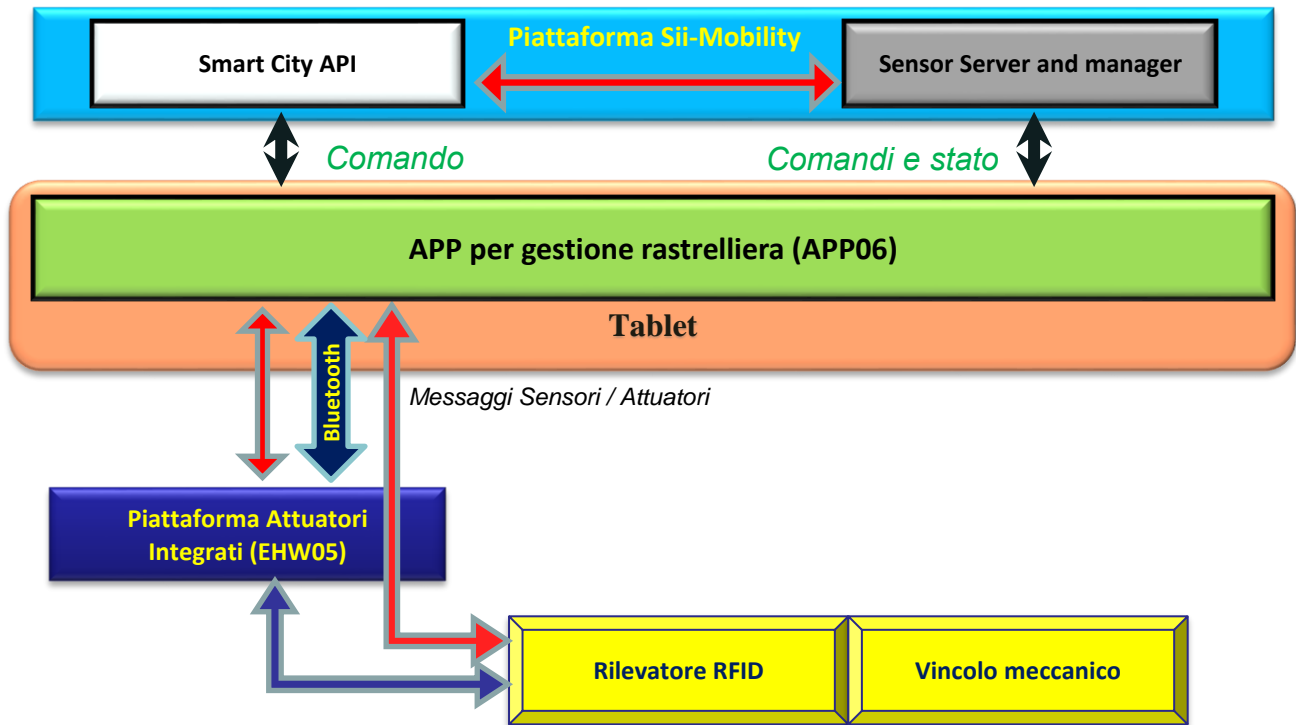
Figura 13 : Architettura generale della Rastrelliera Intelligente
