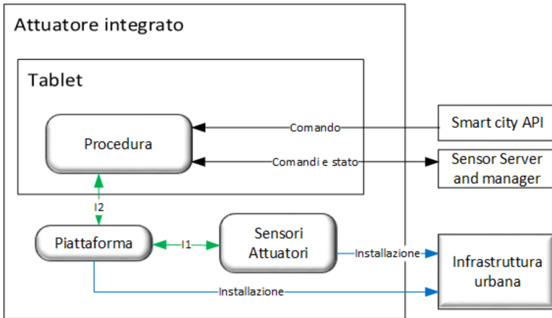
Figura 5 : Struttura comune - diagramma di contesto
