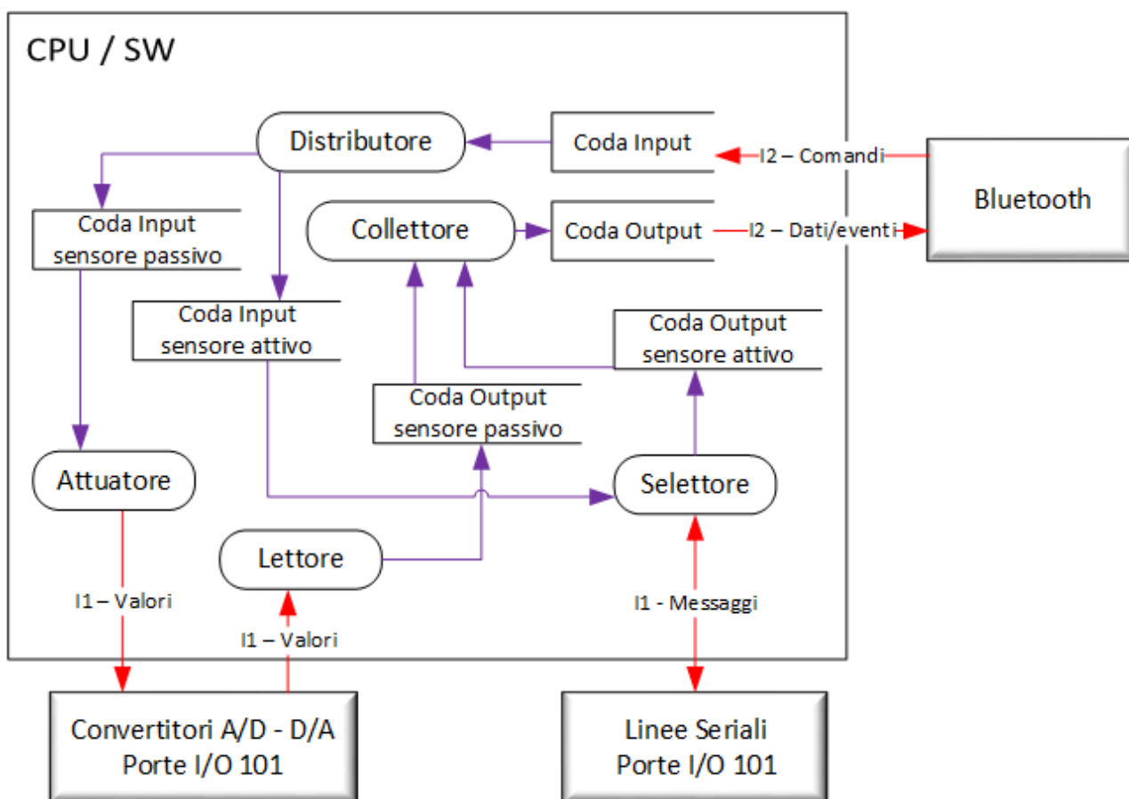
Figura 7 : Architettura di base del software
