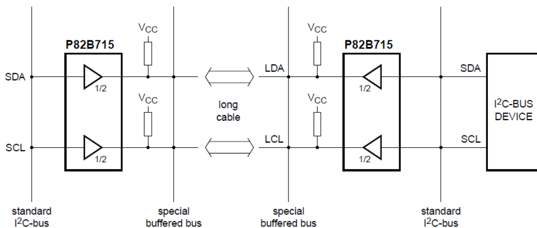
Figura 21 : CHIP P82B715 per estendere il bus I^2C
