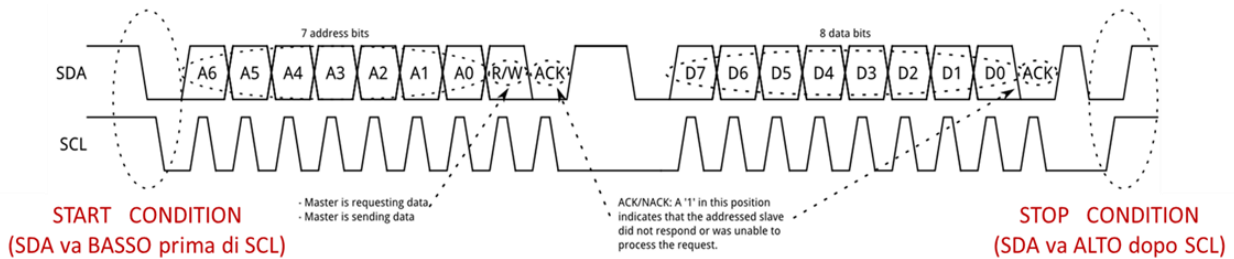
Figura 18 : comunicazione sul bus I 2 C (indirizzo slave + data)
