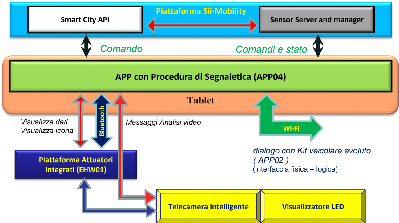
Figura 9 : Architettura generale del Segnale Dinamico
