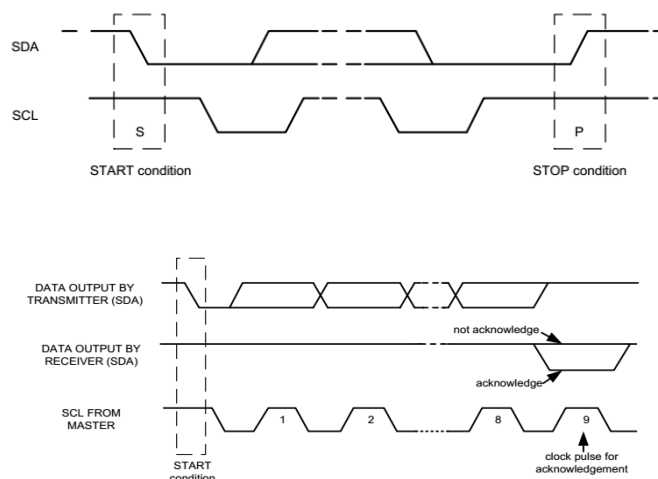
Figura 17 : definizione della fase di START/STOP, ACKNOWLEDGE sul bus I^2C
