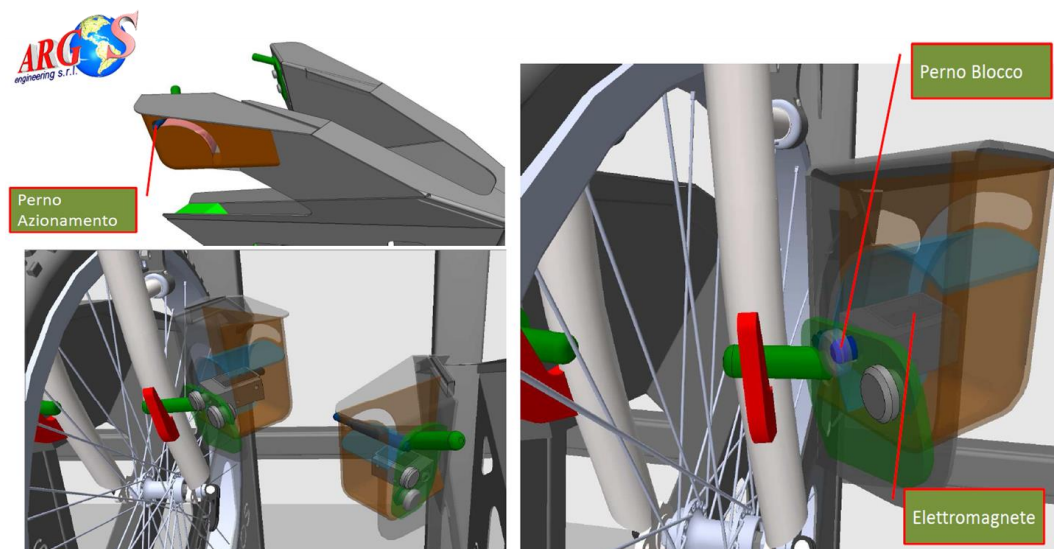
Figura 22 : perno azionamento con intervento esterno (Sx) e elettromagnete dotato di bobina che permette lo sblocco mediante applicazione di una tensione di 12 V (Dx)
