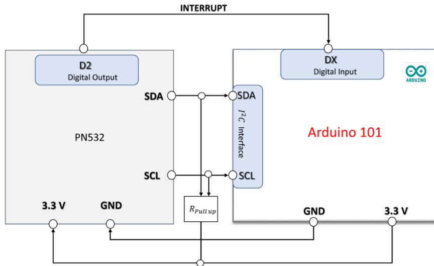
Figura 20 : Comunicazione tra RFID Reader e motherboard (da sviluppare per ogni stallo)
