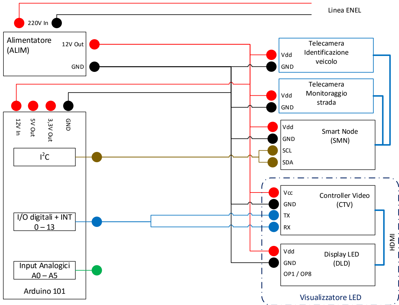
Figura 10 : Schema generale del Segnale Dinamico
