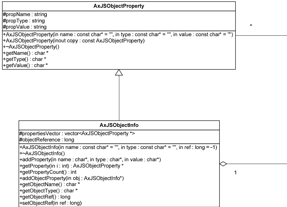
AxJSDebugDataType Class Diagram
